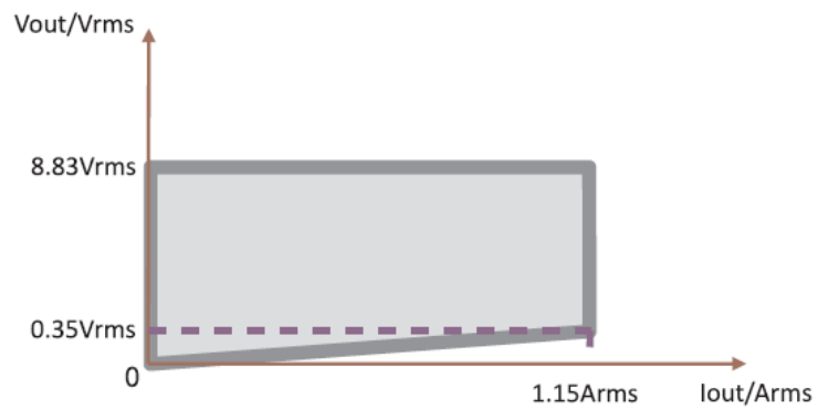
交流工作区域 (25°C, Sine, Freq=100kHz)
