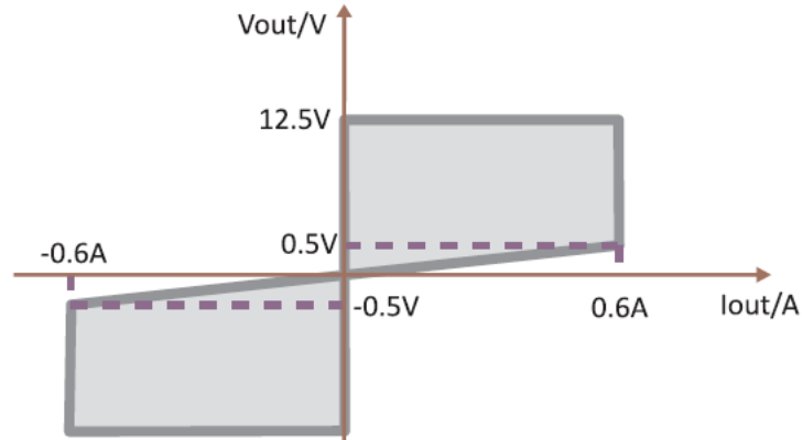
直流工作区域 (25°C, Freq ≤ 50Hz)
